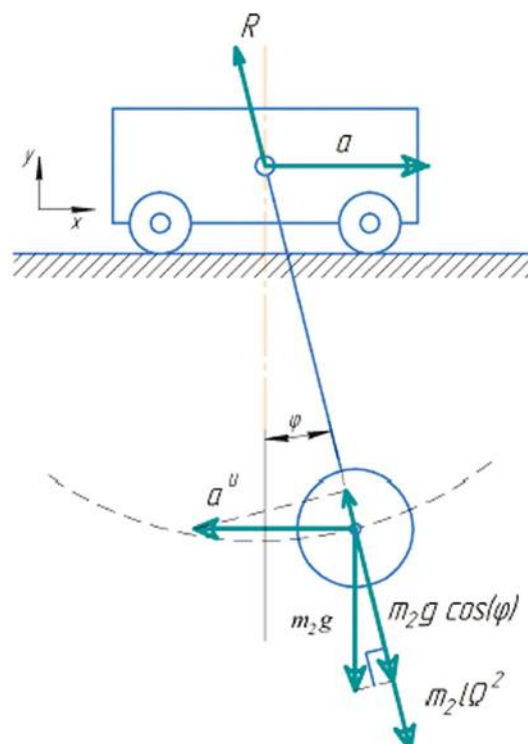
Рис. 1. Расчетная модель мостового крана
