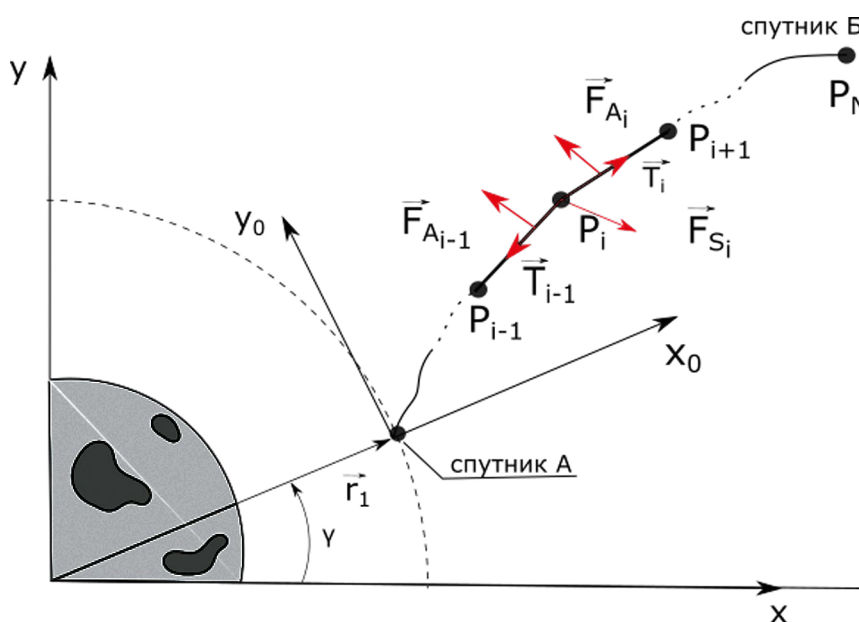
Рис. 1. Механическая система
