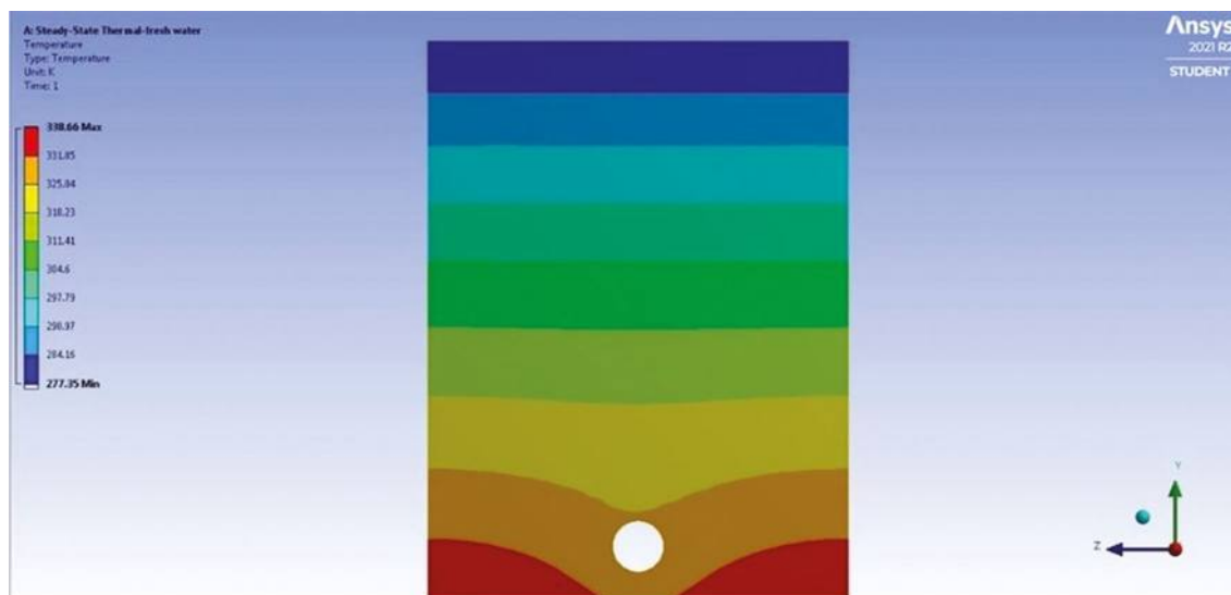
Рис. 2. Распределение температур в пруду с пресной водой. Максимальная температура: 338,66 К; минимальная температура: 277,25 К
