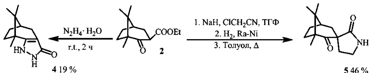
Рис. 2. Синтез гетероциклических производных целевого \beta -кетоефира
