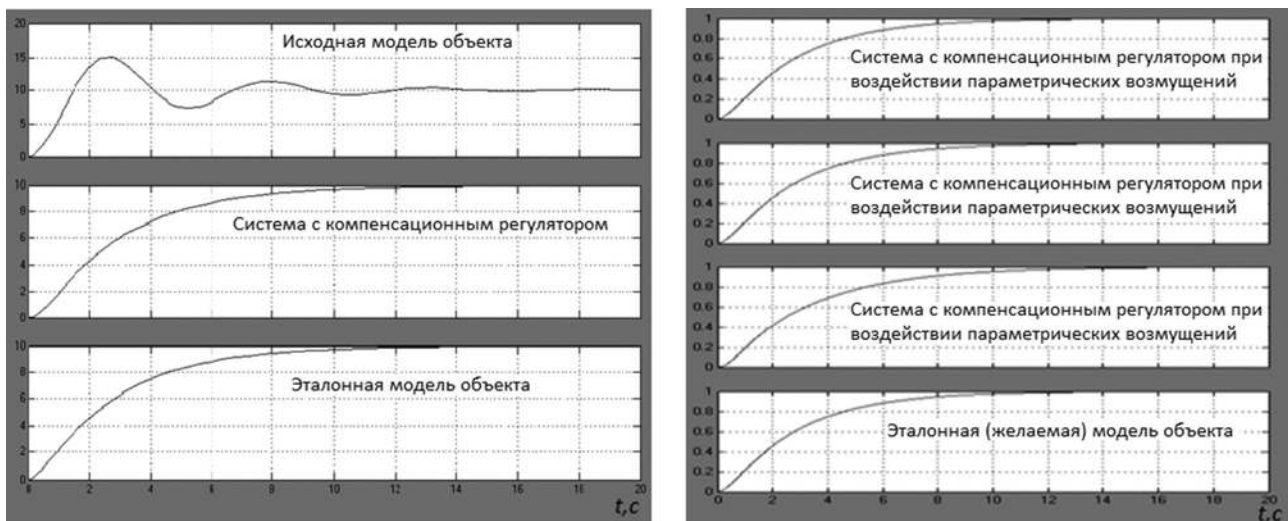
Рис. 3. Результаты моделирования: а — без возмущающего воздействия; б — при воздействии различных параметрических возмущений
