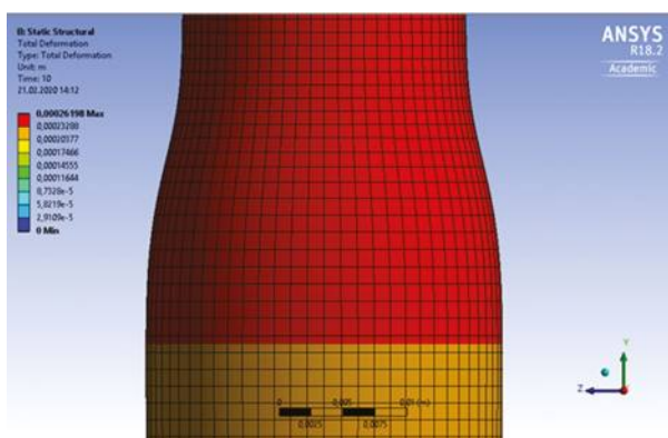
Рис. 3. Деформационная картина на стыке двух сред в тигеле реактора
