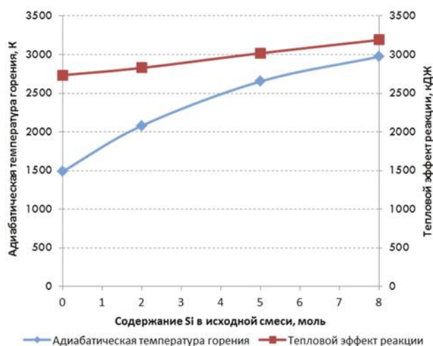
Рис. 2. Зависимость адиабатической температуры реакции и теплового эффекта реакции от содержания Si в системе « \text{Si}-\text{Na}_2\text{SiF}_6-4\text{NaN}_3 »
