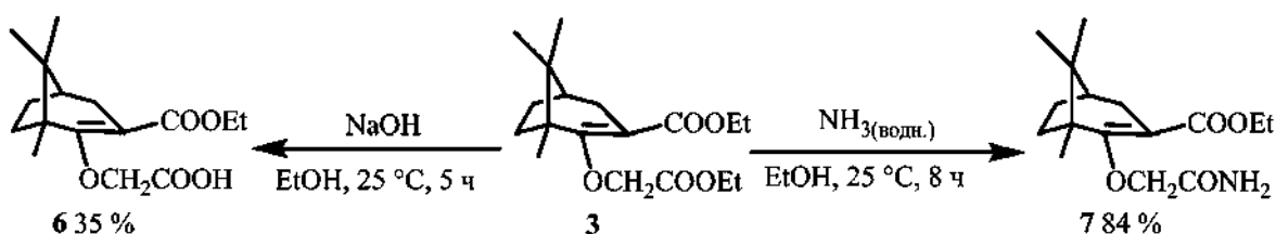
Рис. 3. Синтез карбоновой кислоты и амида
