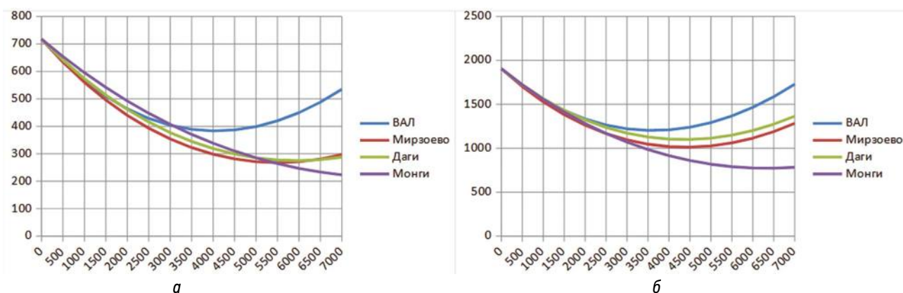
Рис. 3. Графики потерь активной (а) и реактивной (б) мощности в сети в зависимости от мощности, выдаваемой системой аккумуляции
