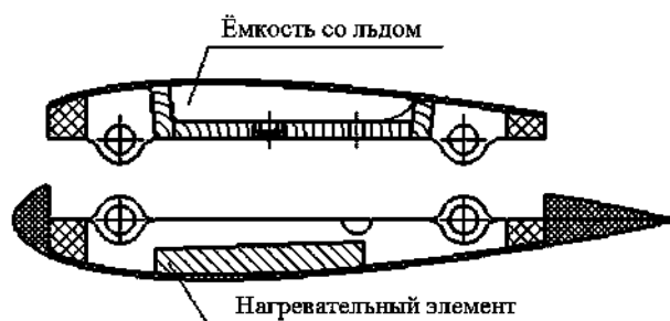
Рис. 1. Сечение экспериментальной модели
