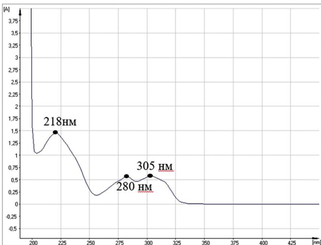
Рис. Электронный спектр глицина
